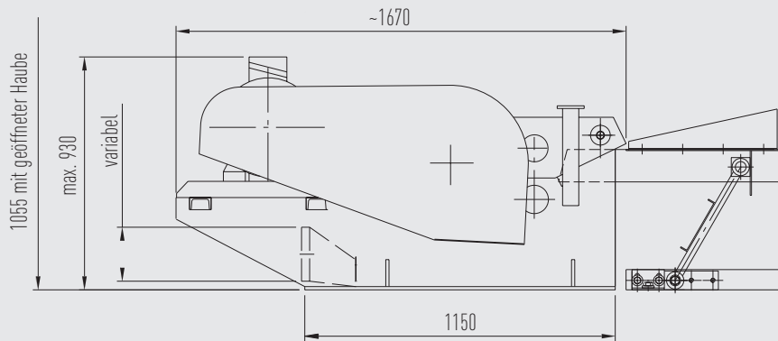
Seitenansicht
