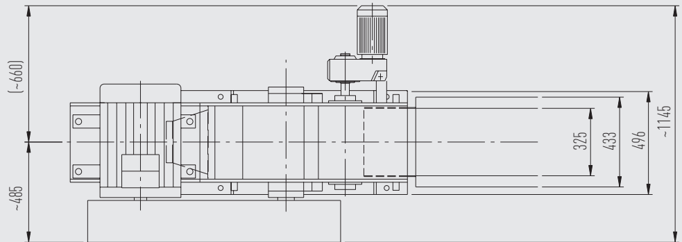
Draufsicht
