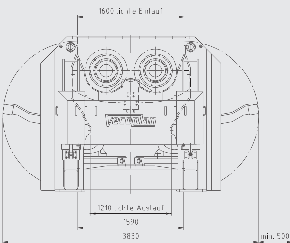
Frontansicht
