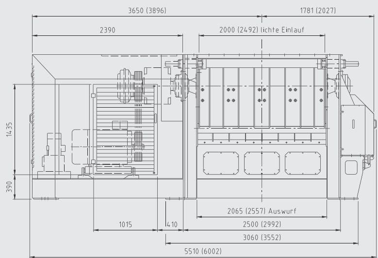
Seitenansicht
