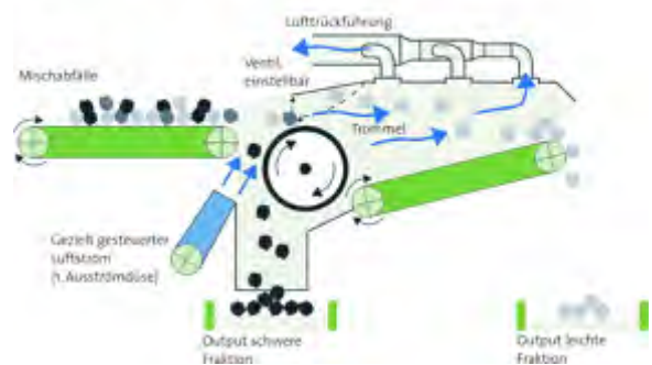
Funktionsschema des Single-Drum Separator.
